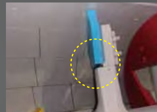
パドルとアームの間をフラット形状にし付着を抑制しました
