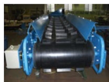
◎横サン付ベルト コンベヤを傾斜で使用する時 中寄ベルトでは転がる時
