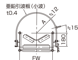
点検用風防カバー (常時点検が必要な箇所に取付けます)
