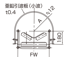
固定用風防カバー
