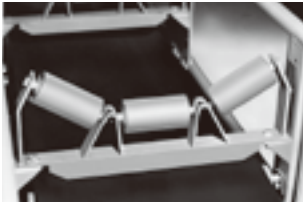
3槽式アイドラ
