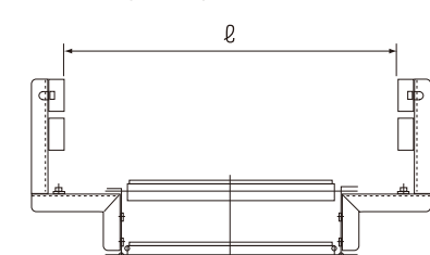
MR・50-4-M・HDS-SK (横サン付ベルト、スカート、落下防止板) (オプション)
