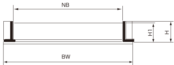
傾斜直線ライン用 (I型) に使用
