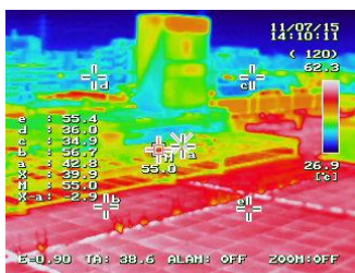
何も塗布していないコンクリート製の屋上
