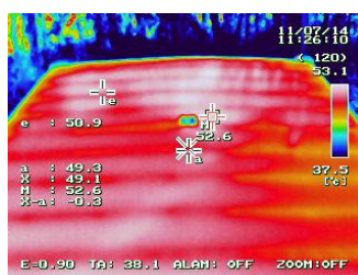
他社製遮熱塗料を塗布した鋼板製の屋根
