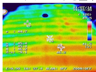
タフコートを塗布した鋼板製の屋根
